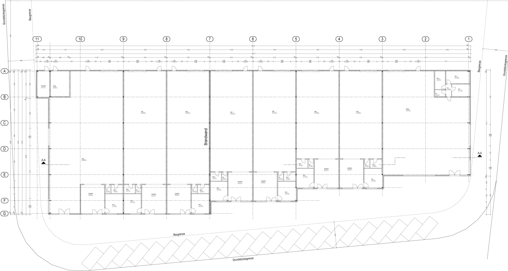
Grundriss
